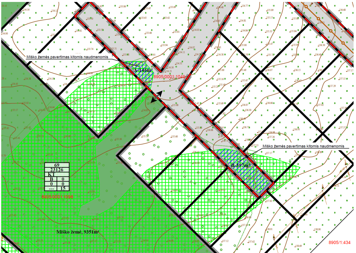
Pagrindinio brėžinio fragmentas
