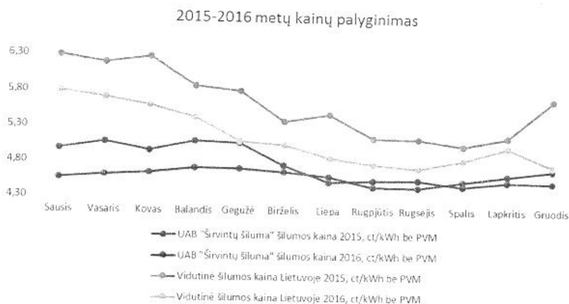
1 pav. Bendrovės šilumos kainų kitimo dinamika 2015-2016 metais ir jų palyginimas su šalies vidutine kaina 2015- 2016 metais
